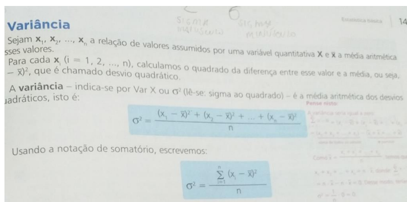
Figura 20: Fórmula da variância do livro didático
