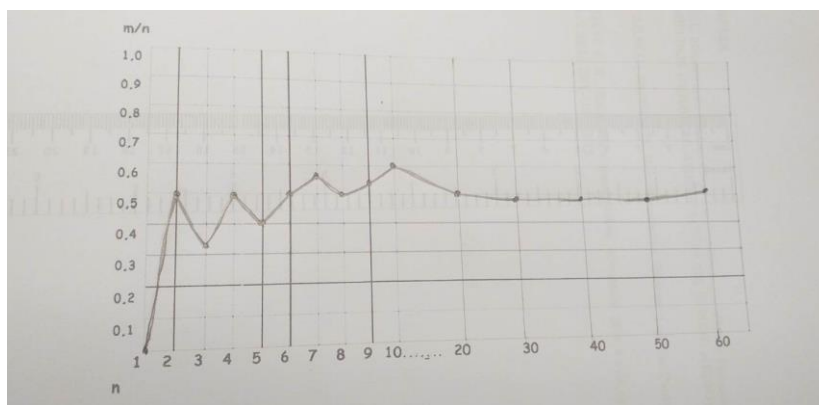
(b) Gráfico de Poisson Fonte: Dados da pesquisa
