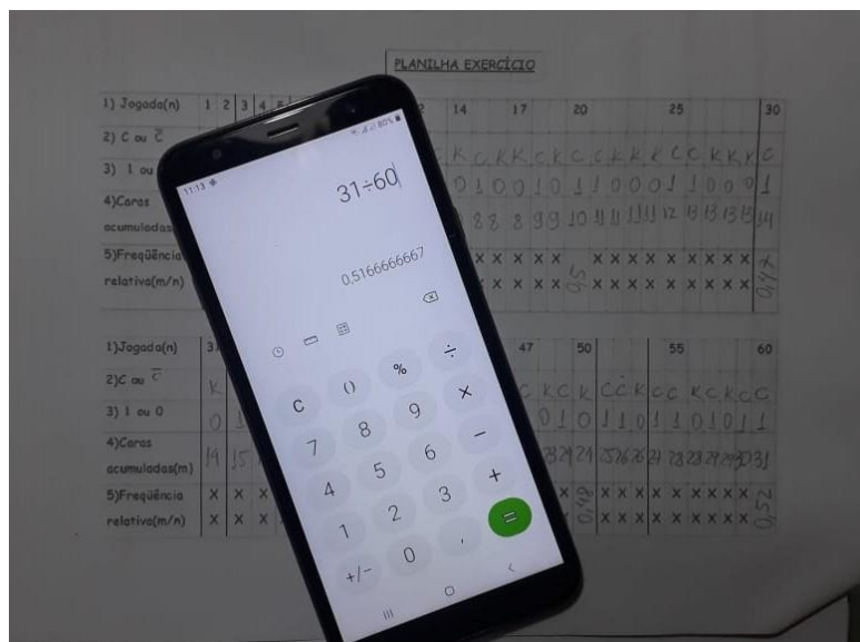
Figura 17: Uso do celular como calculadora na oficina
