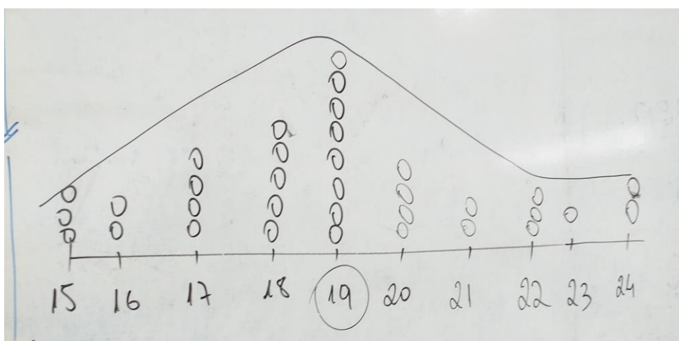
Figura 23: Gráfico de pontos da medida do palmo da mão
