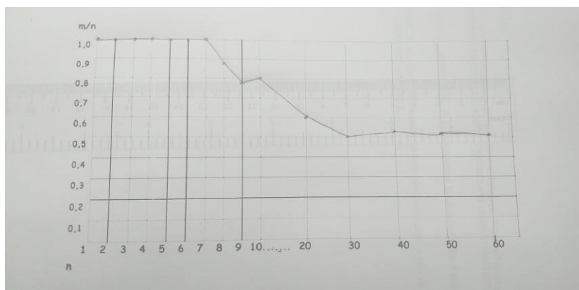
(a) Gráfico de Kolmogorov
